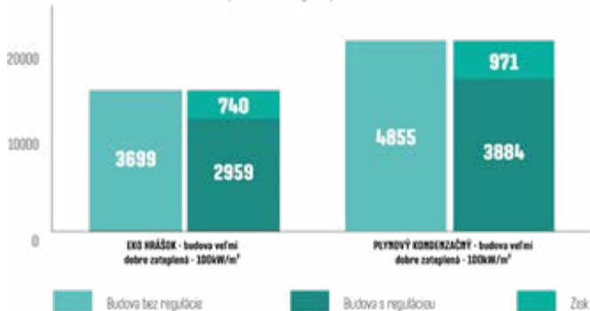
Náklady na vykurovanie bez regulácie a s reguláciou pre budovu s objemnou plochou 1000m 2
