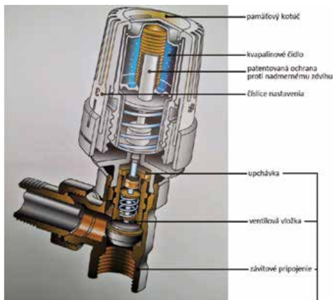
Termostatický ventil OVENTROP
