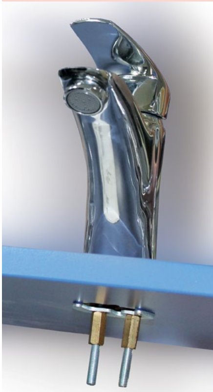
Batéria je prichytená krátkymi alebo dlhými maticami
